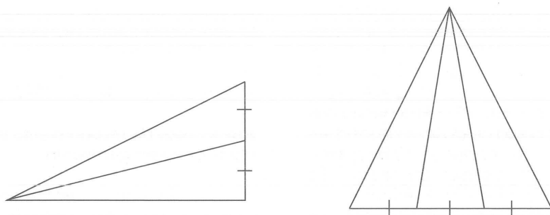
Figura 2. Construcciones de la bisección y la trisección de un ángulo basadas en asunciones erróneas de linealidad.
